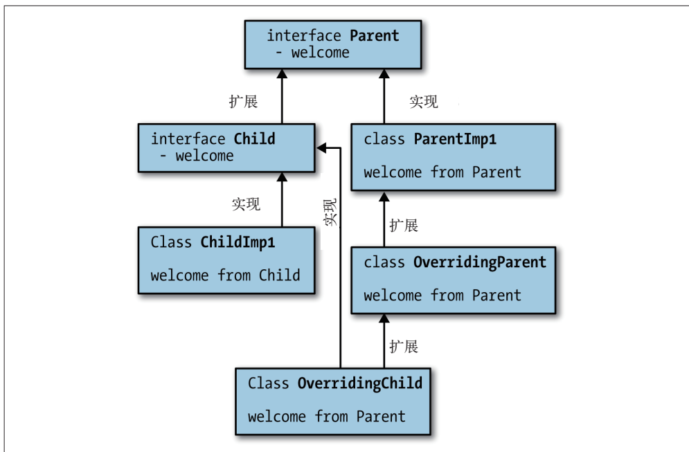
图 4-5: 完整的继承体系图
