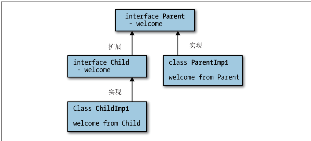
图 4-4: 类继承体系图
