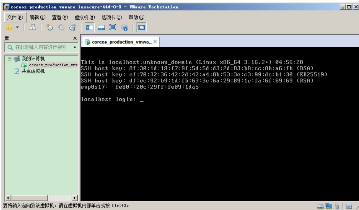
图 1.23.5.3 - 登录 CoreOS
