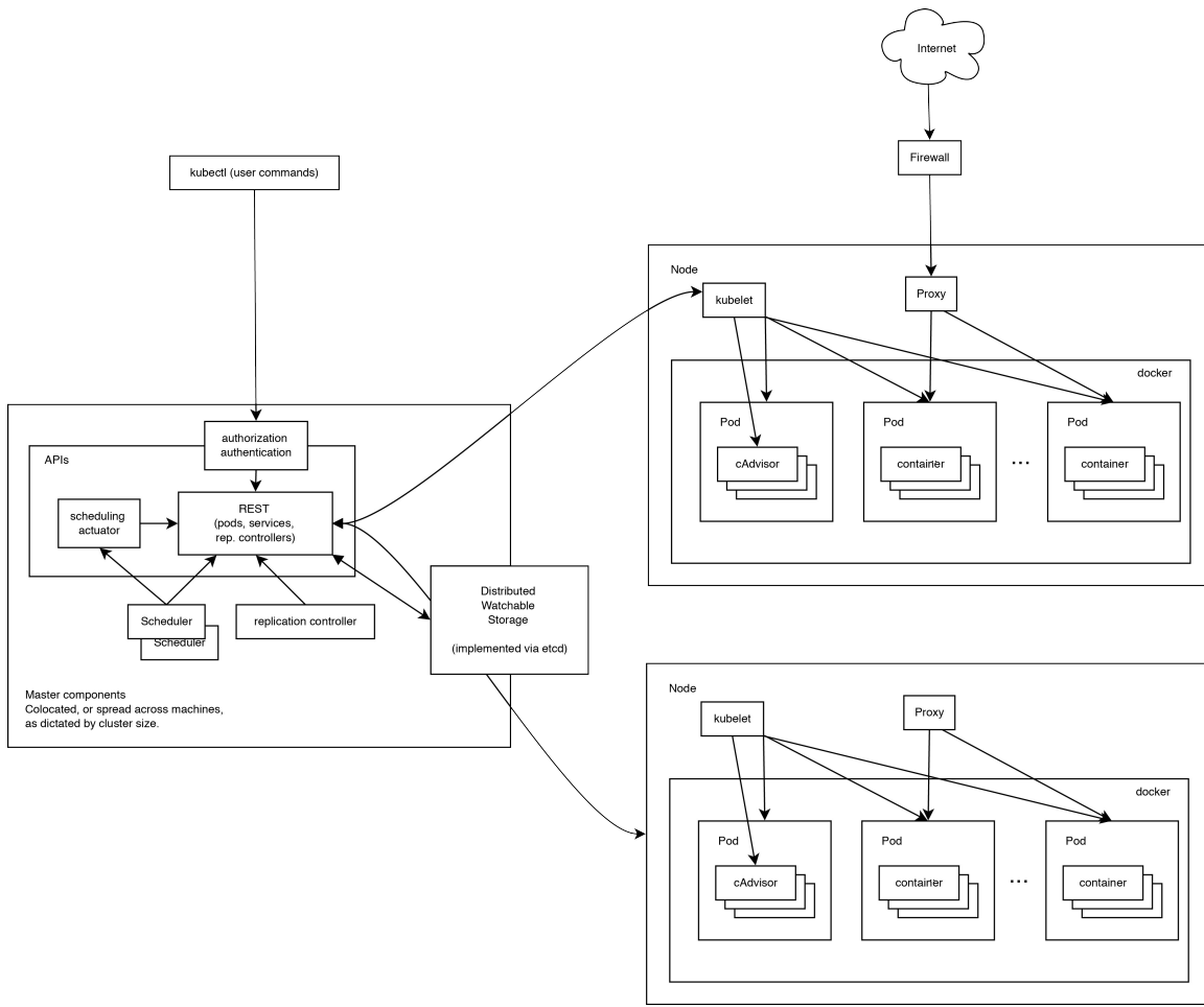
图 1.20.5.1 - Kubernetes 架构
